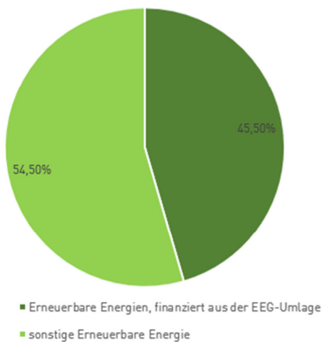
Strommix - SENECloud
