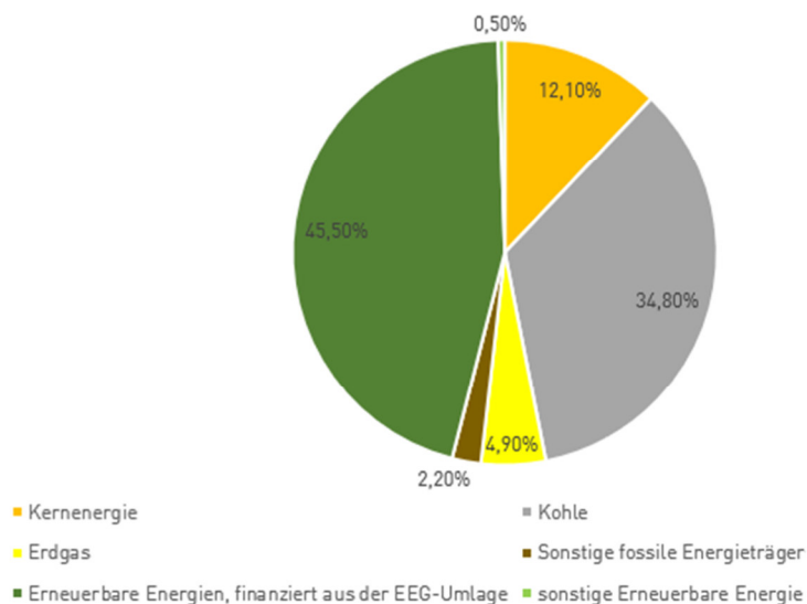
Strommix - Deutschland
